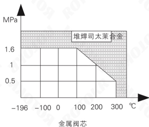
阀内件温度-压力曲线 (图四)
