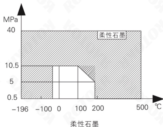
填料温度-压力曲线 (图六)
